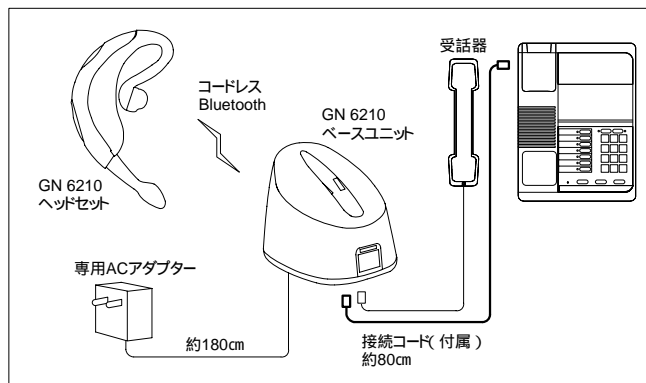
電話機接続の例
